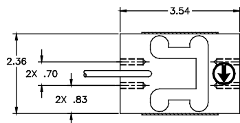
6 kg dimensions
